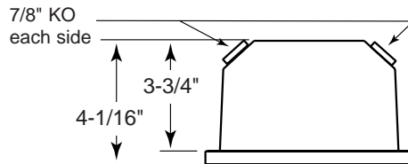
FC SL401 Open Die Cast Face
